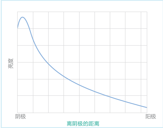
亮度
