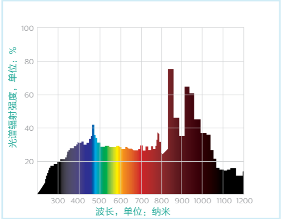
光谱分布
