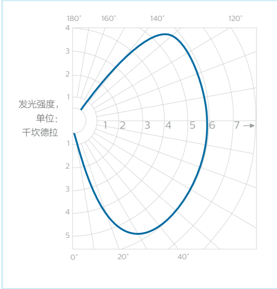
发光强度
